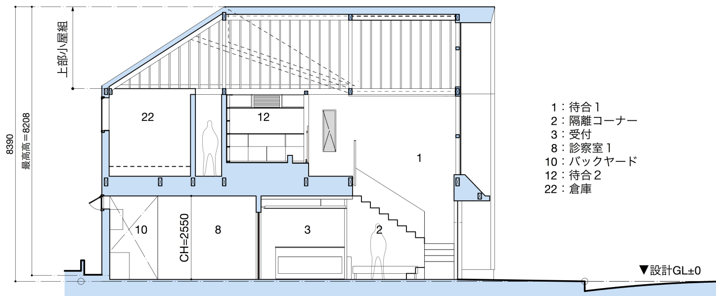
B-B 断面図
