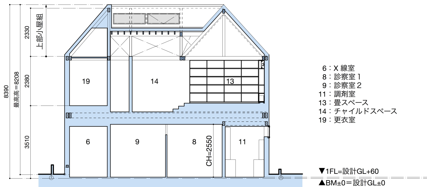
A-A 断面図
