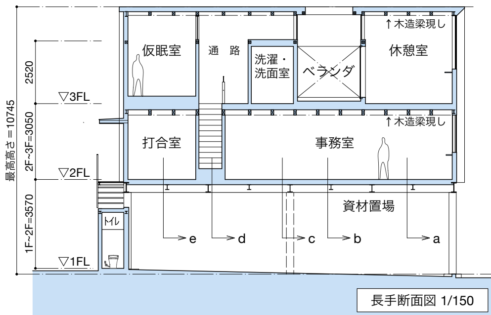
断面図 1/150
