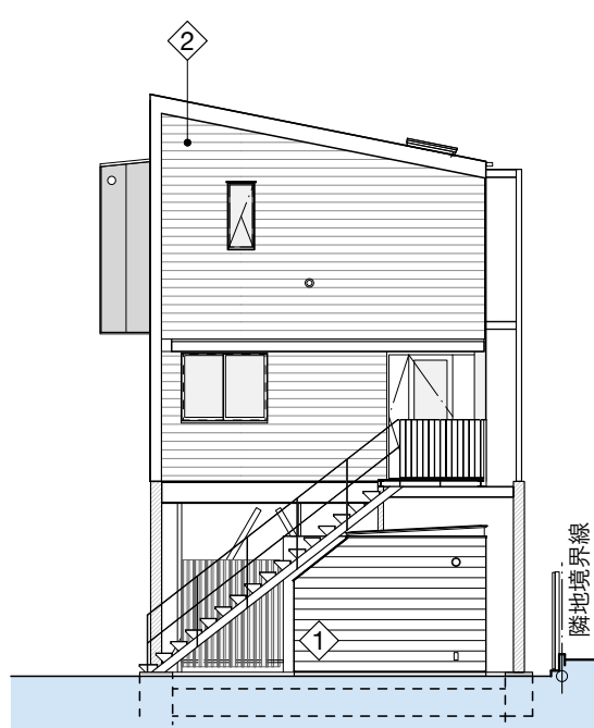
南立面図 1/150
