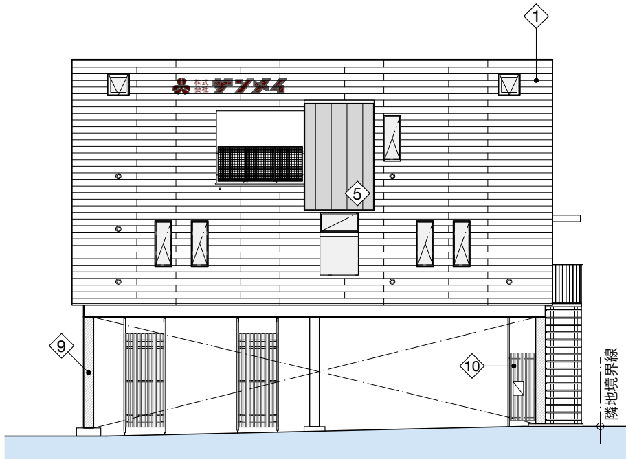
西立面図 1/150
