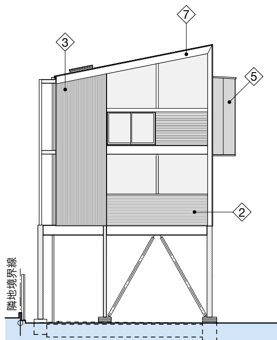
北立面図 1/150
