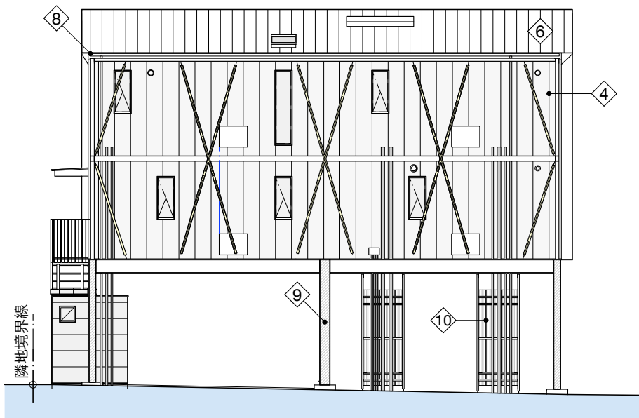
東立面図 1/150
