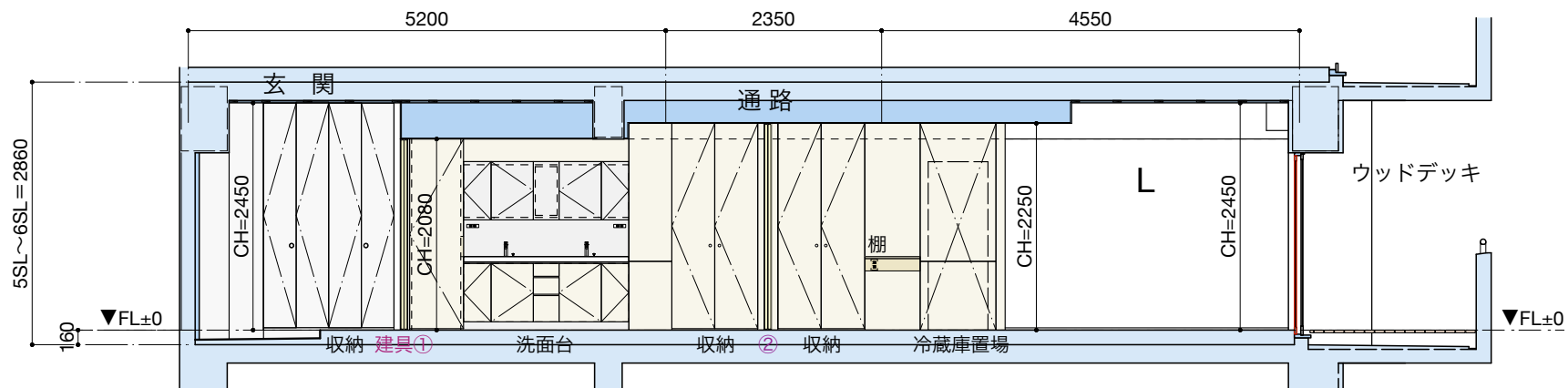
A-A 断面図：生活動線の展開図
