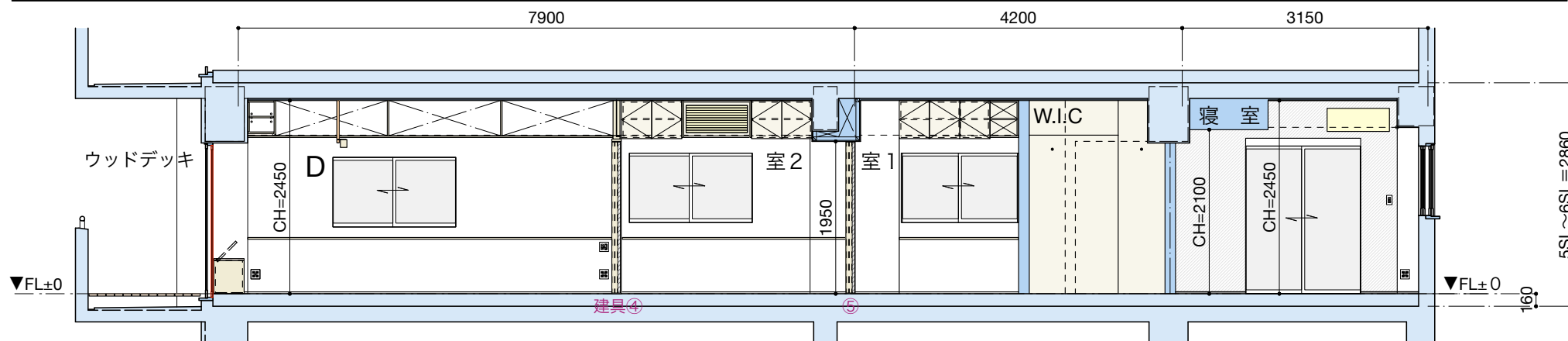
B-B 断面図：空間動線の展開図
